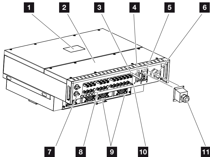
Fig. 9 : Onduleur PIKO CI 50/60 (vue extérieure)
