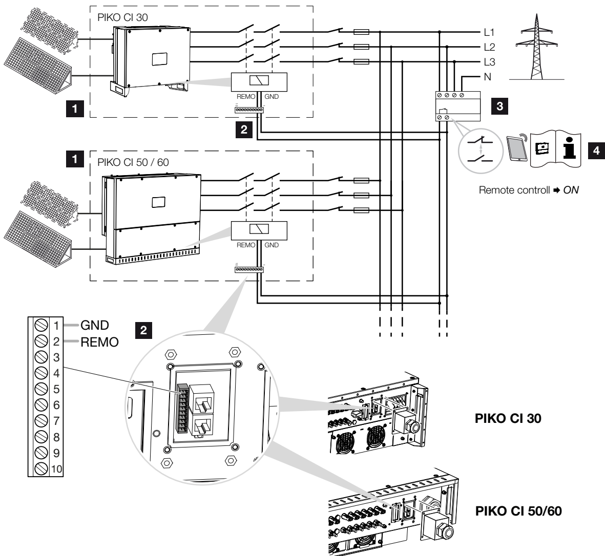
Fig. 27 : Protection centrale du réseau et de l'installation avec disjoncteur de couplage
