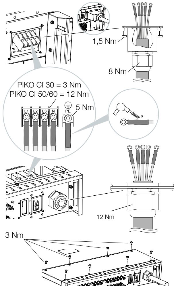
Fig. 17 : Isoler la connexion AC
