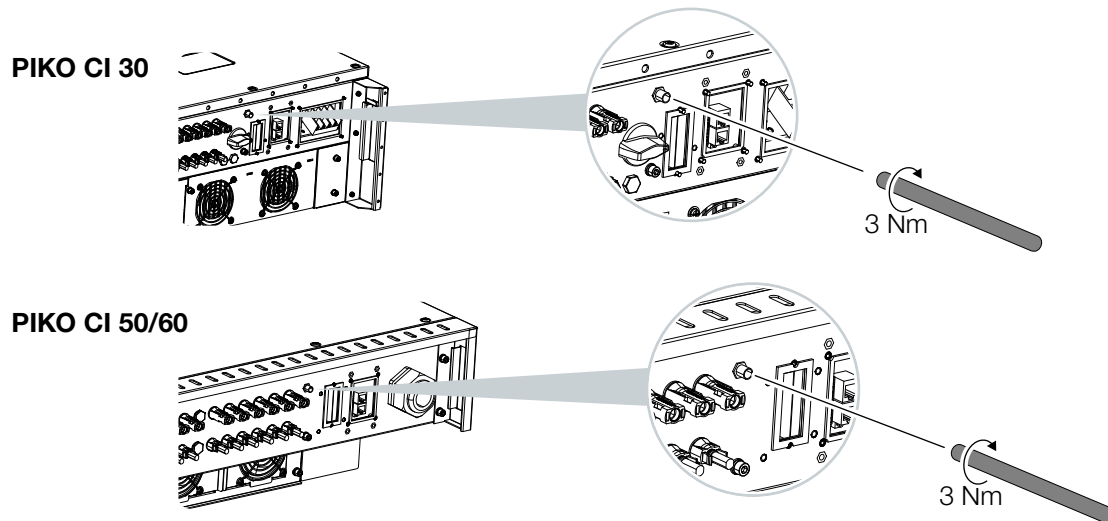
Fig. 20 : Monter l'antenne Wi-Fi
