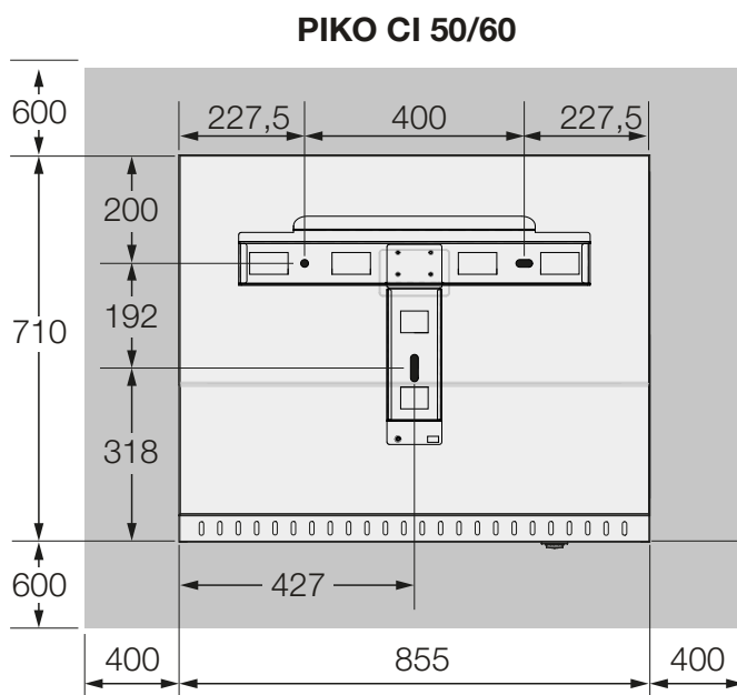
Fig. 12 : Dimensions de montage avec support
