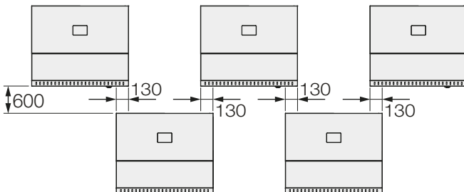
Fig. 13 : Plusieurs onduleurs côte à côte
