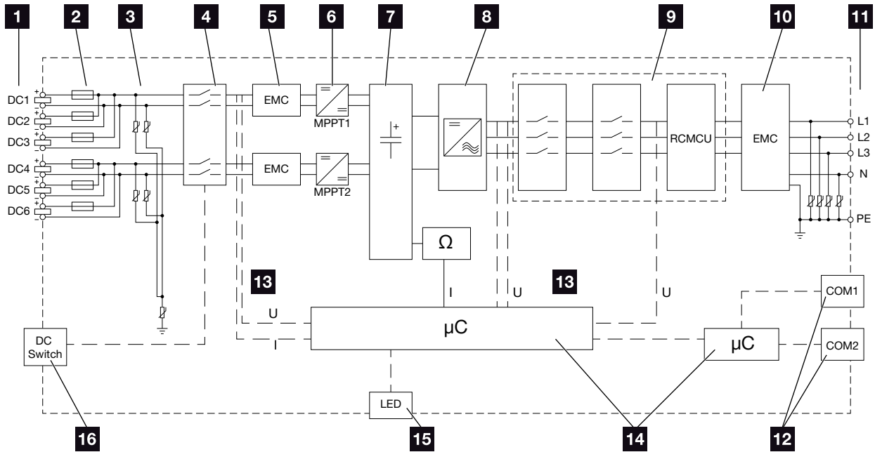
Fig. 34 : Schéma fonctionnel PIKO CI 30
