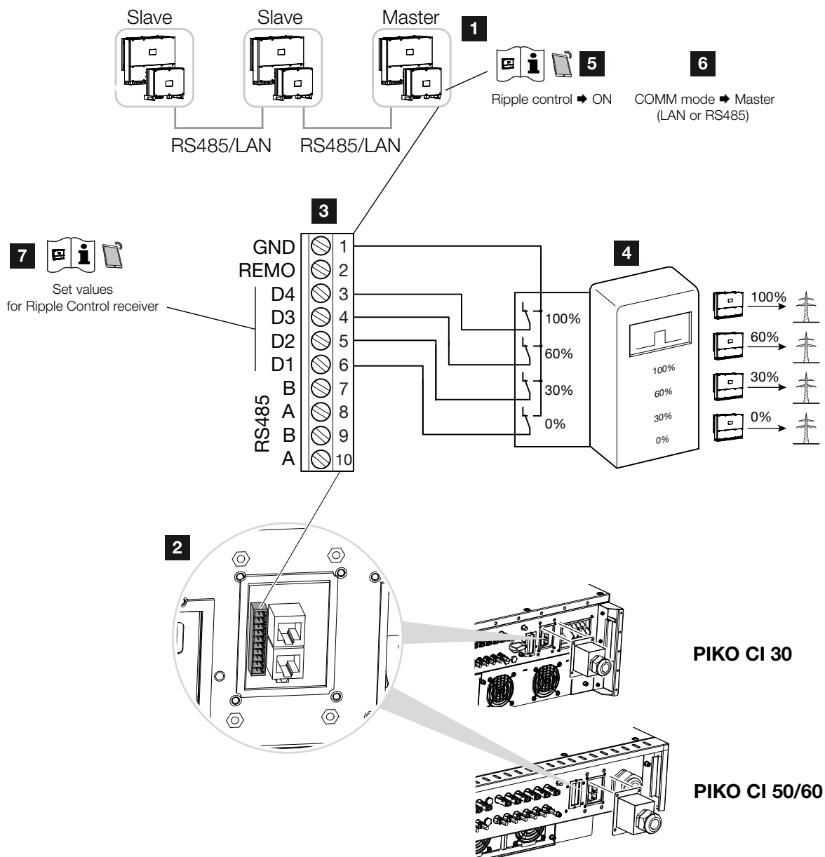
Fig. 29 : Raccordement du récepteur centralisé
