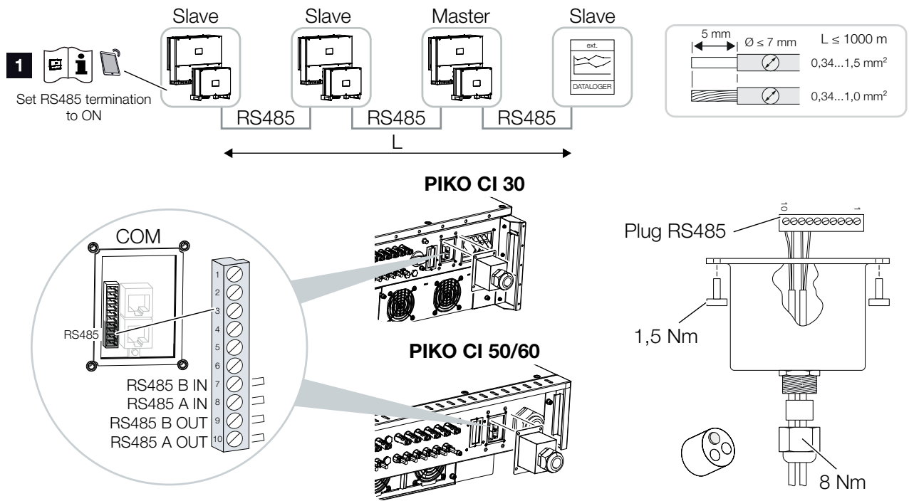
Fig. 23 : Connecter l'onduleur avec un câble RS485
