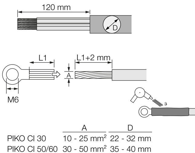
Fig. 16 : Préparer le câble AC
