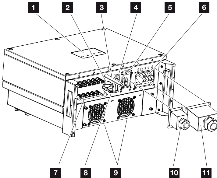
Fig. 8 : Onduleur PIKO CI 30 (vue extérieure)
