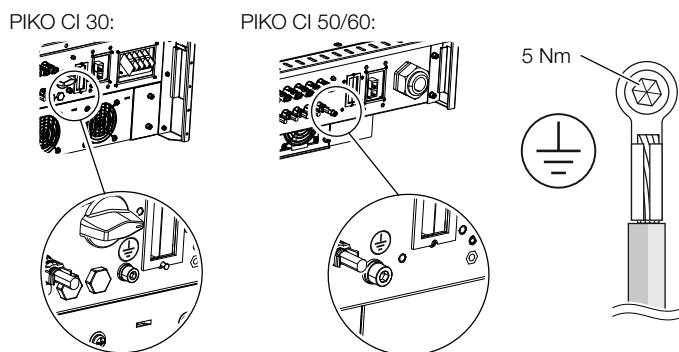
Fig. 18 : Raccordement PE externe propre à chaque pays
