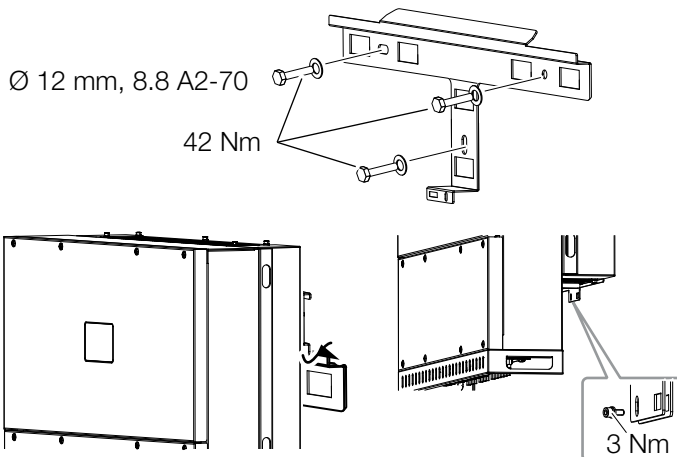
Fig. 14 : Installation de l'onduleur PIKO CI
