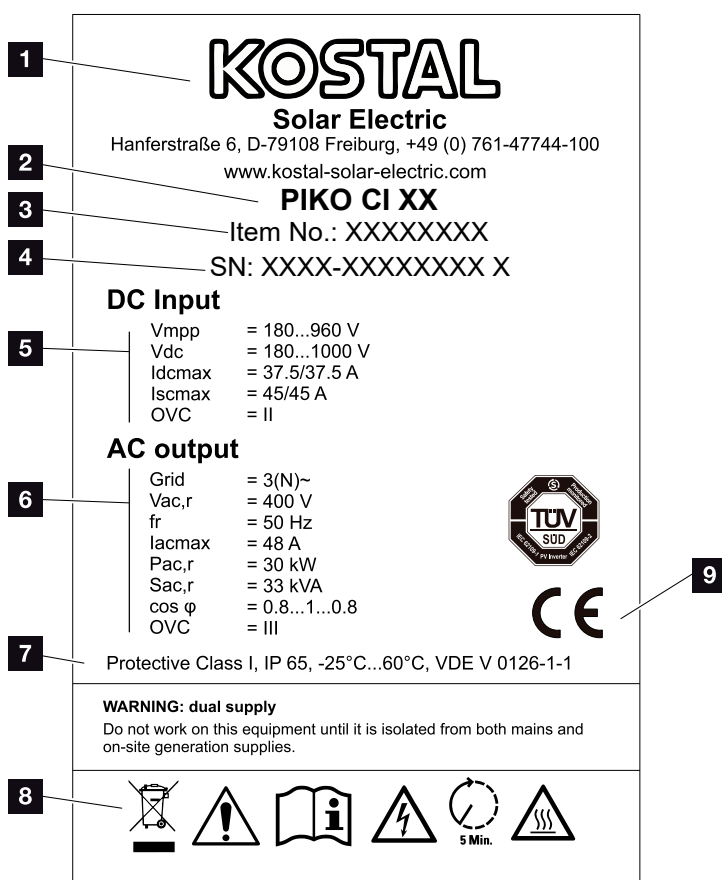
Fig. 37 : Plaque signalétique
