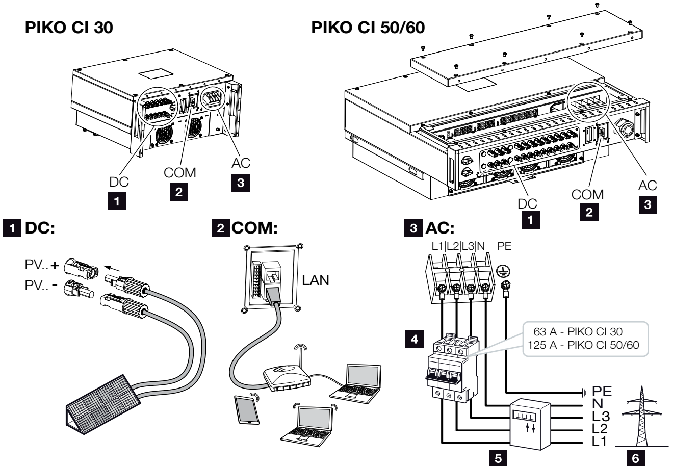
Fig. 15 : Aperçu des raccordements électriques
