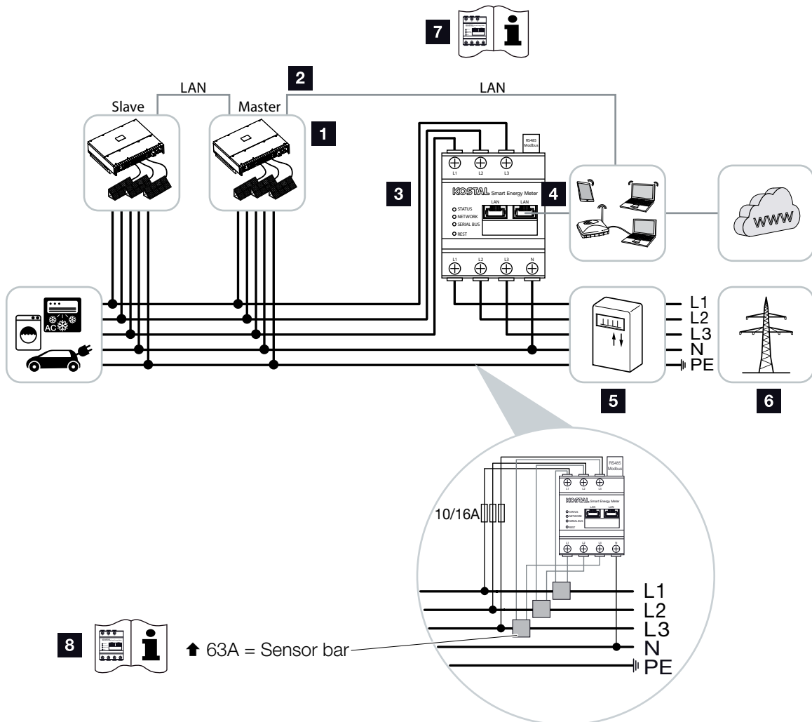
Fig. 25 : Schéma de câblage compteur d'énergie LAN - connexion au réseau
