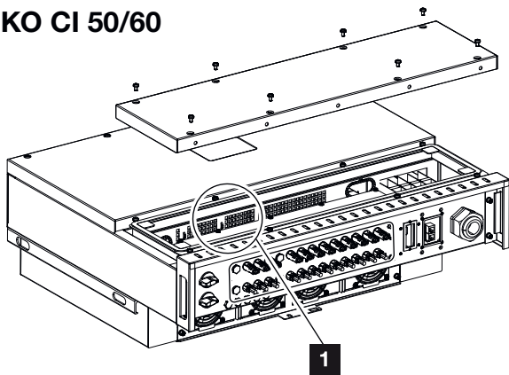
Fig. 33 : Onduleur PIKO CI 50/60 (fusibles PV)
