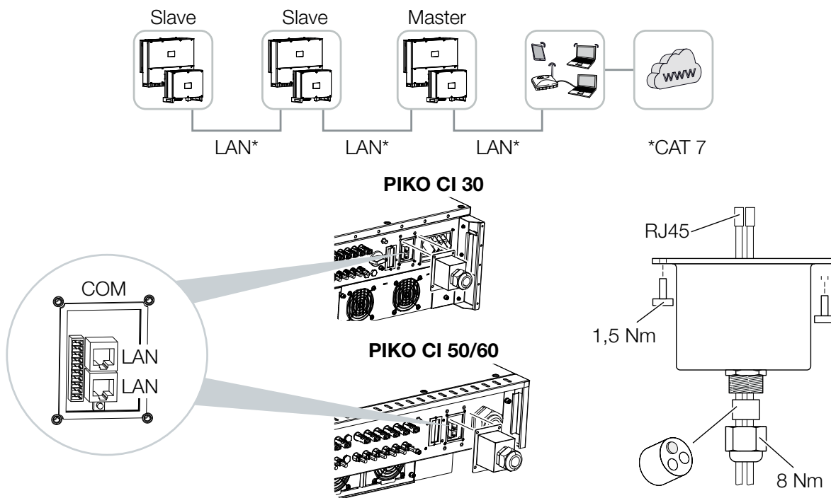
Fig. 22 : Raccorder l'onduleur via le câble LAN/Ethernet
