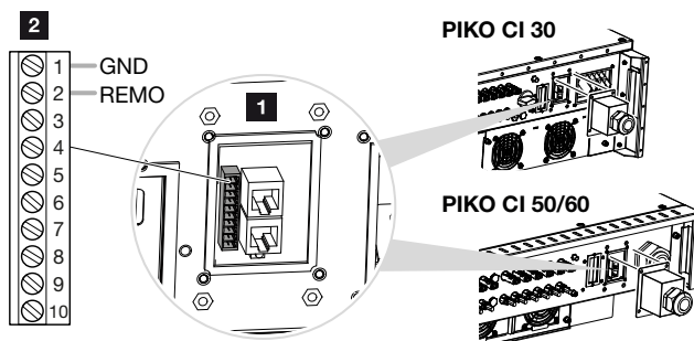
Fig. 28 : Protection centrale de l'installation - Connexion
